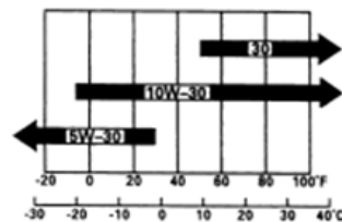
Рисунок 8. Замена масла в двигателе
